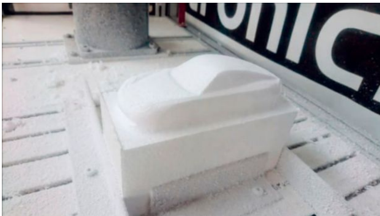
Robotska ćelija je opremljena vretenom za glodanje. Izmena alata na vretenu se radi ručno.
